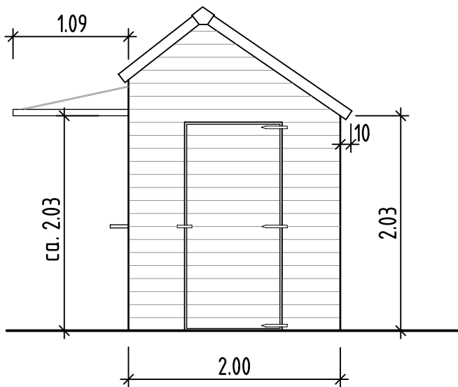
Seitenansicht 1
