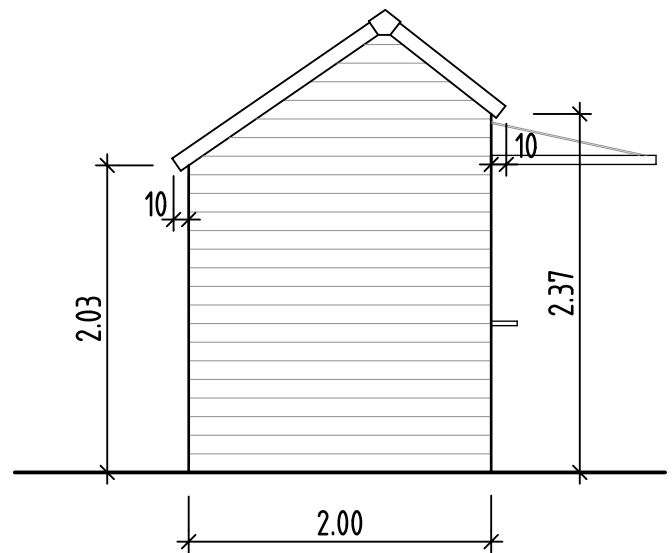
Seitenansicht 2
