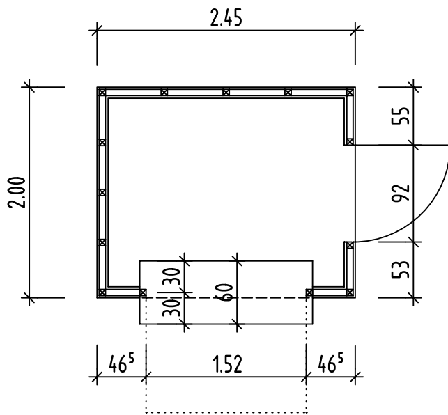
Grundriss
